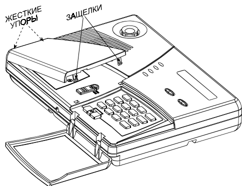
Рисунок 11. Снятие левой крышки
