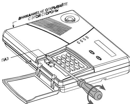
Рисунок 10. Открытие крышки
