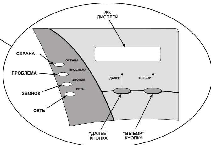
Рисунок 4. Панель управления, кнопки управления и индикаторы
