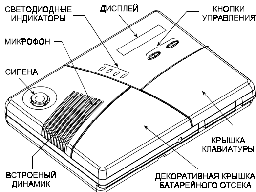
Рисунок 1. Панель управления (с закрытой крышкой)
