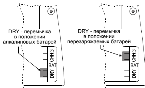
Рисунок 14. Переключатель батарей
